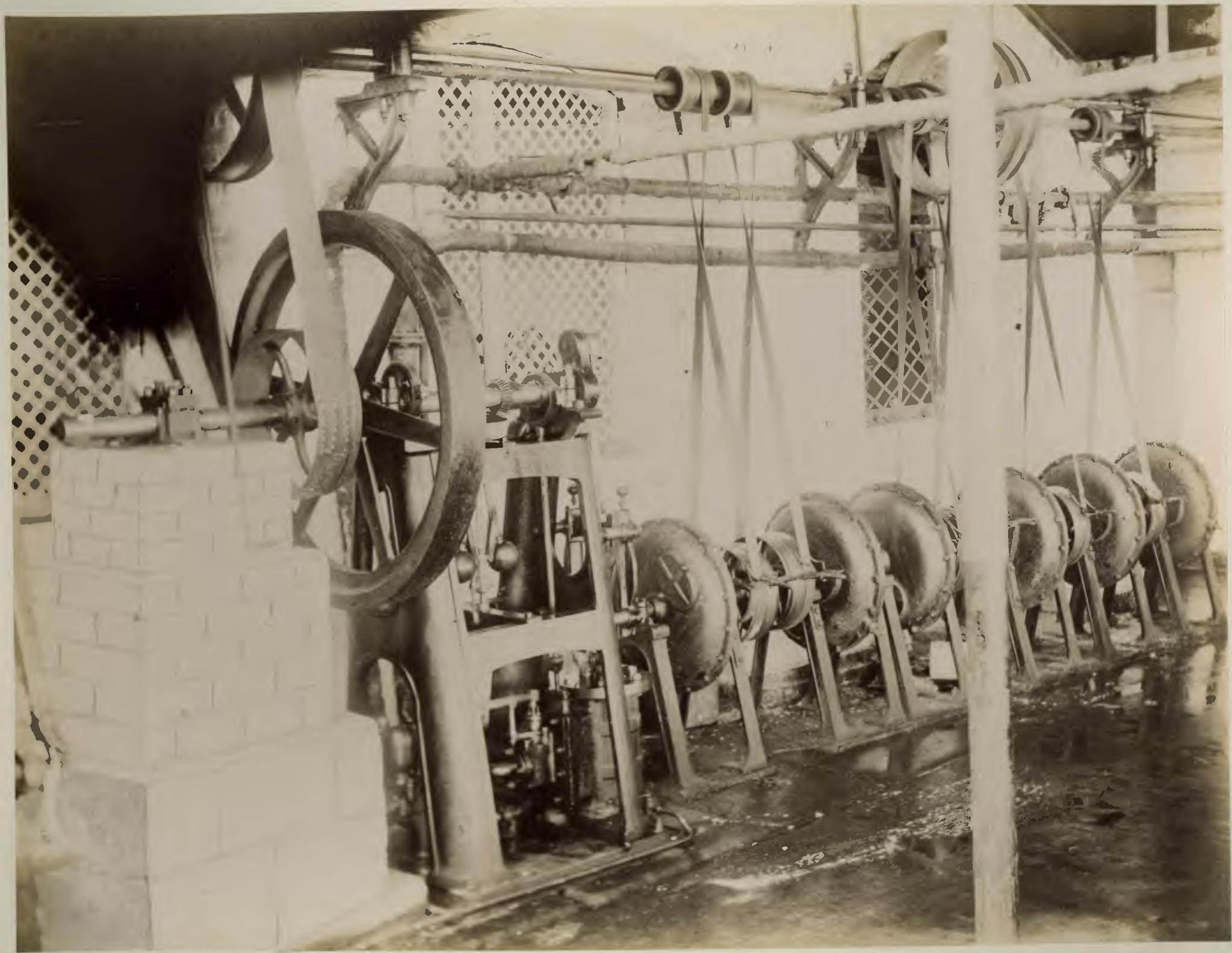
Краскотерные машины. - Machines à broyer les couleurs.
