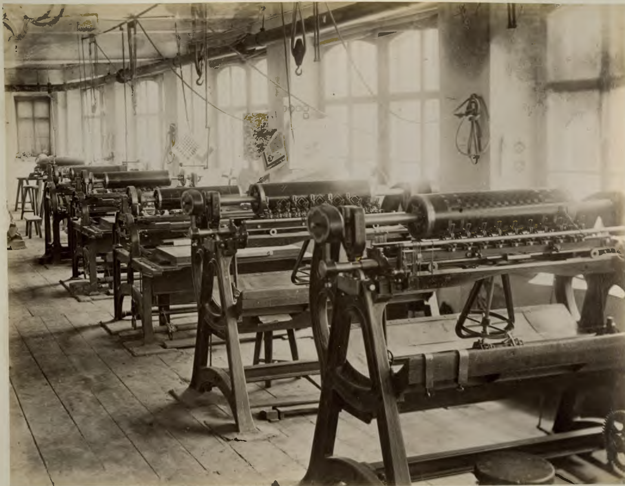
Гравировальные машины пантографы. ~ Machines à graver pantograpbes.
