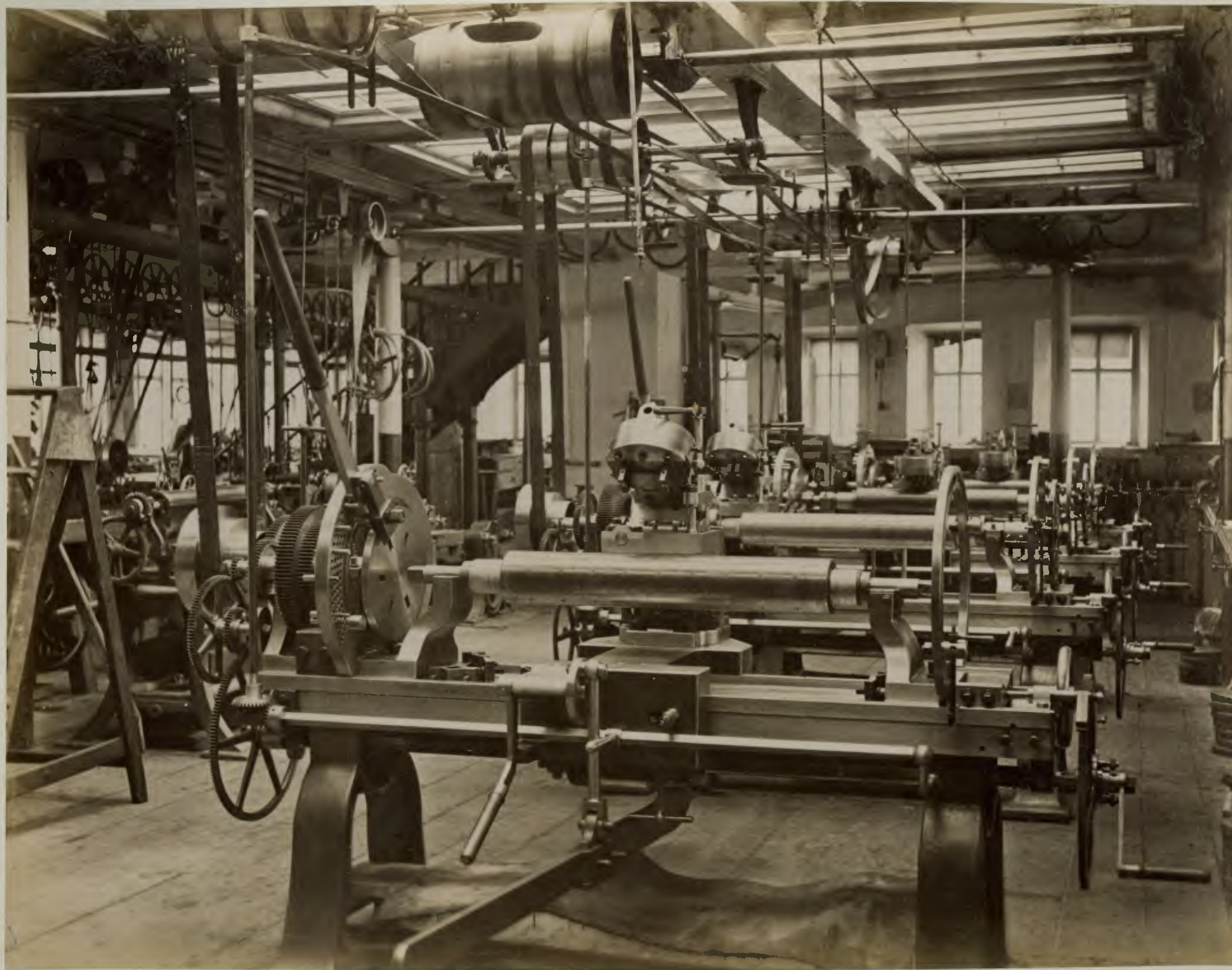
Накаменная машина. ~ Machines à moletter.
