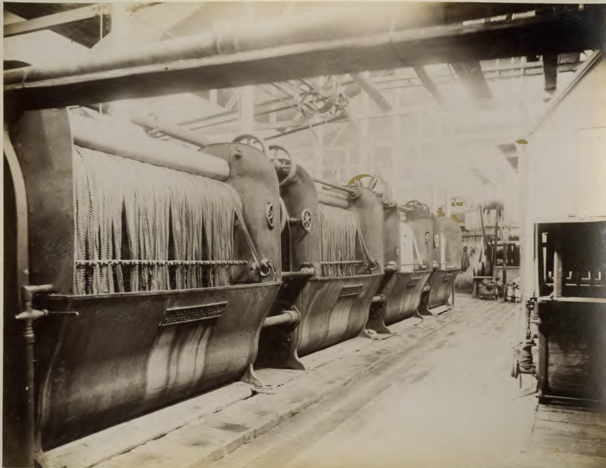
Видъ красильни. - Vue de la teinture.
