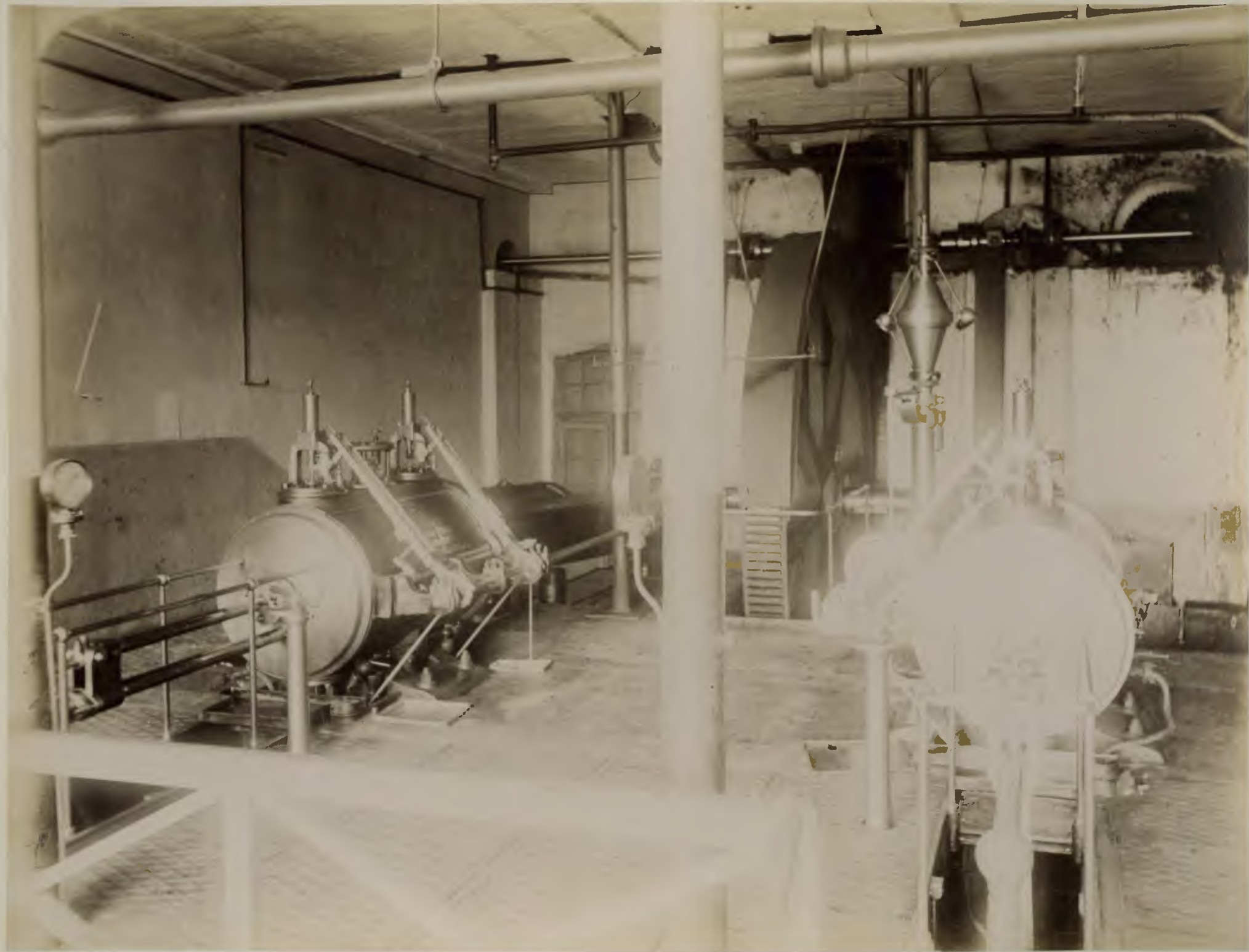
Паровая машина для отбелной и красильной. - Machine à vapeur du Blanchiment et de la Teinture.
