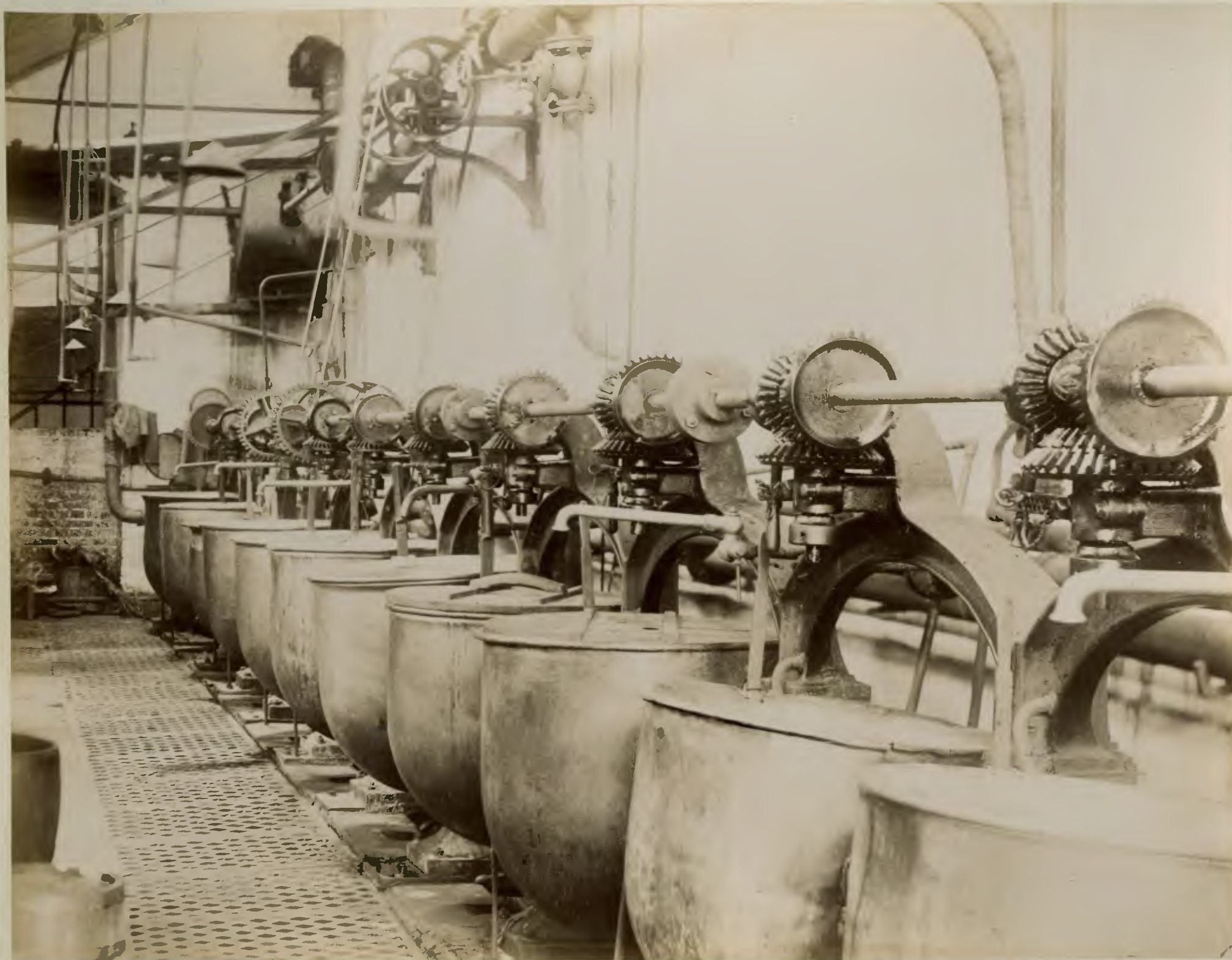
Красковарные котлы ~ Les chaudières à cuire les couleurs.
